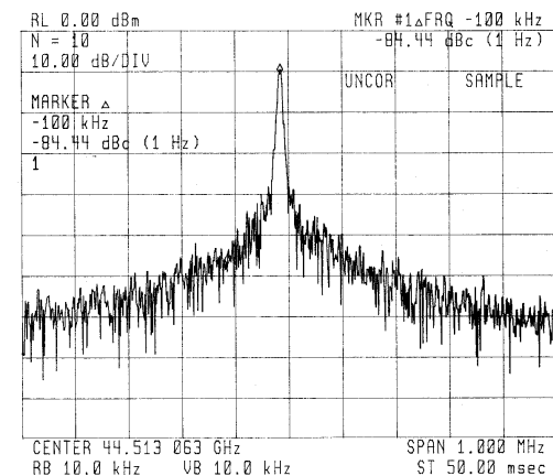
Fig. 15: DRO output spectrum
